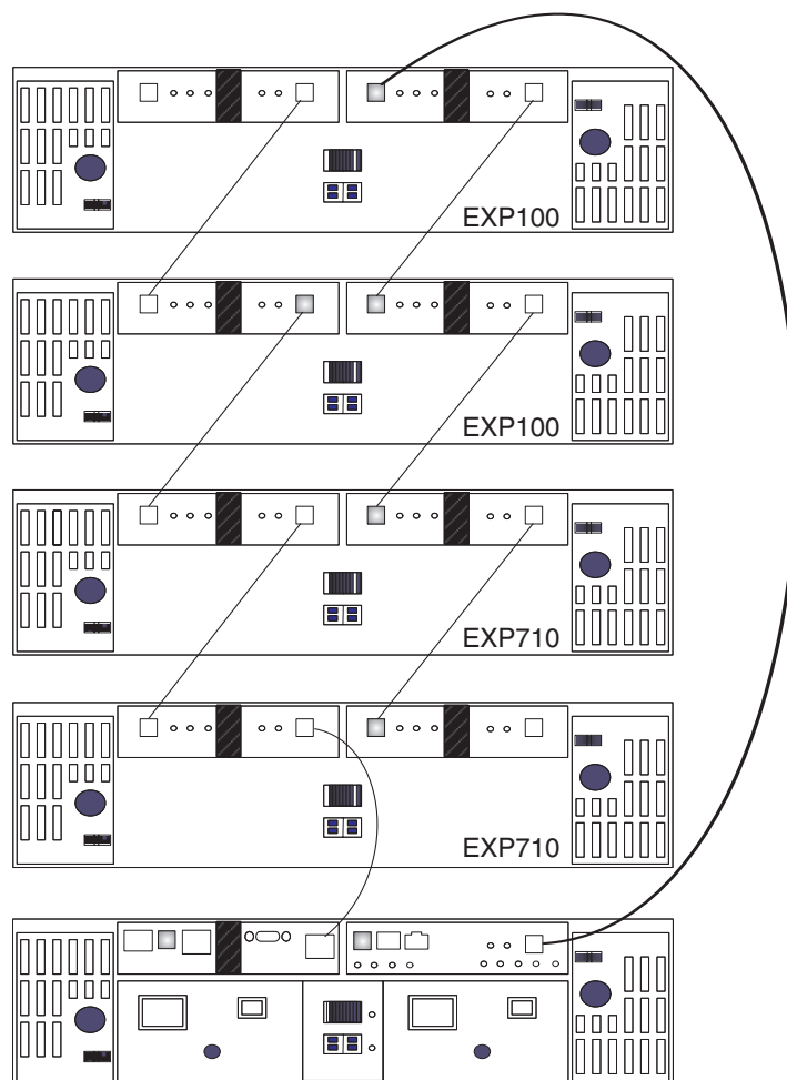
Figura 1. Configuração suportada do loop do gabinete de armazenamento EXP100 e EXP710 (1 de 3)
