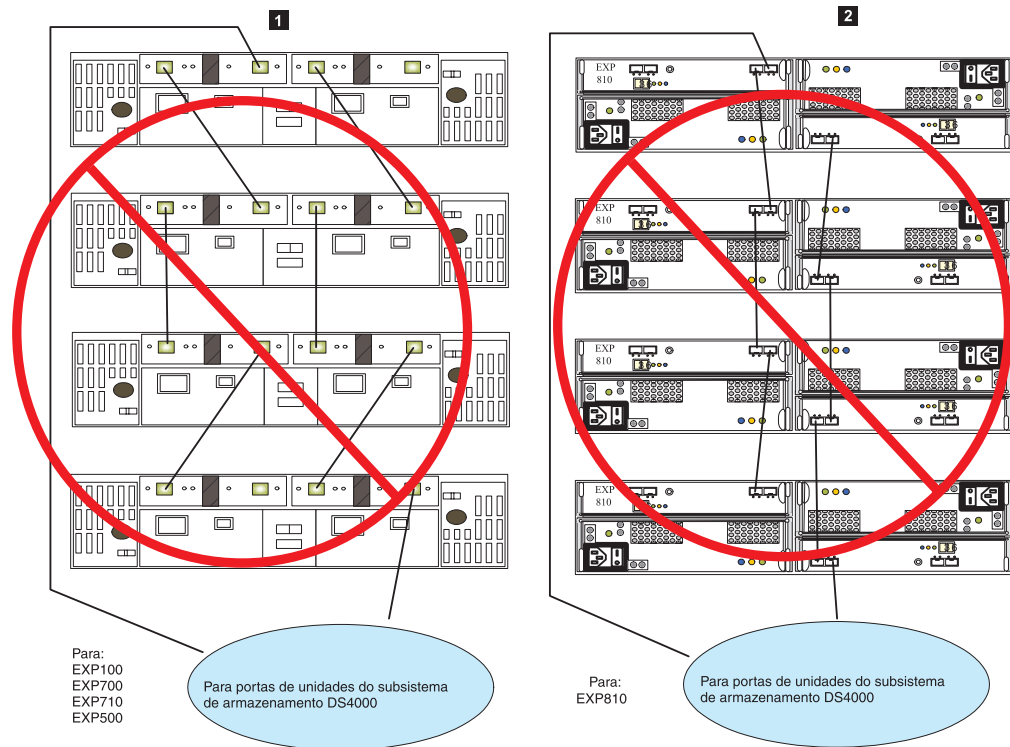
Figura 39. Esquema de loop de cabo não suportado para conexão de dispositivos de armazenamento (2 de 2)
