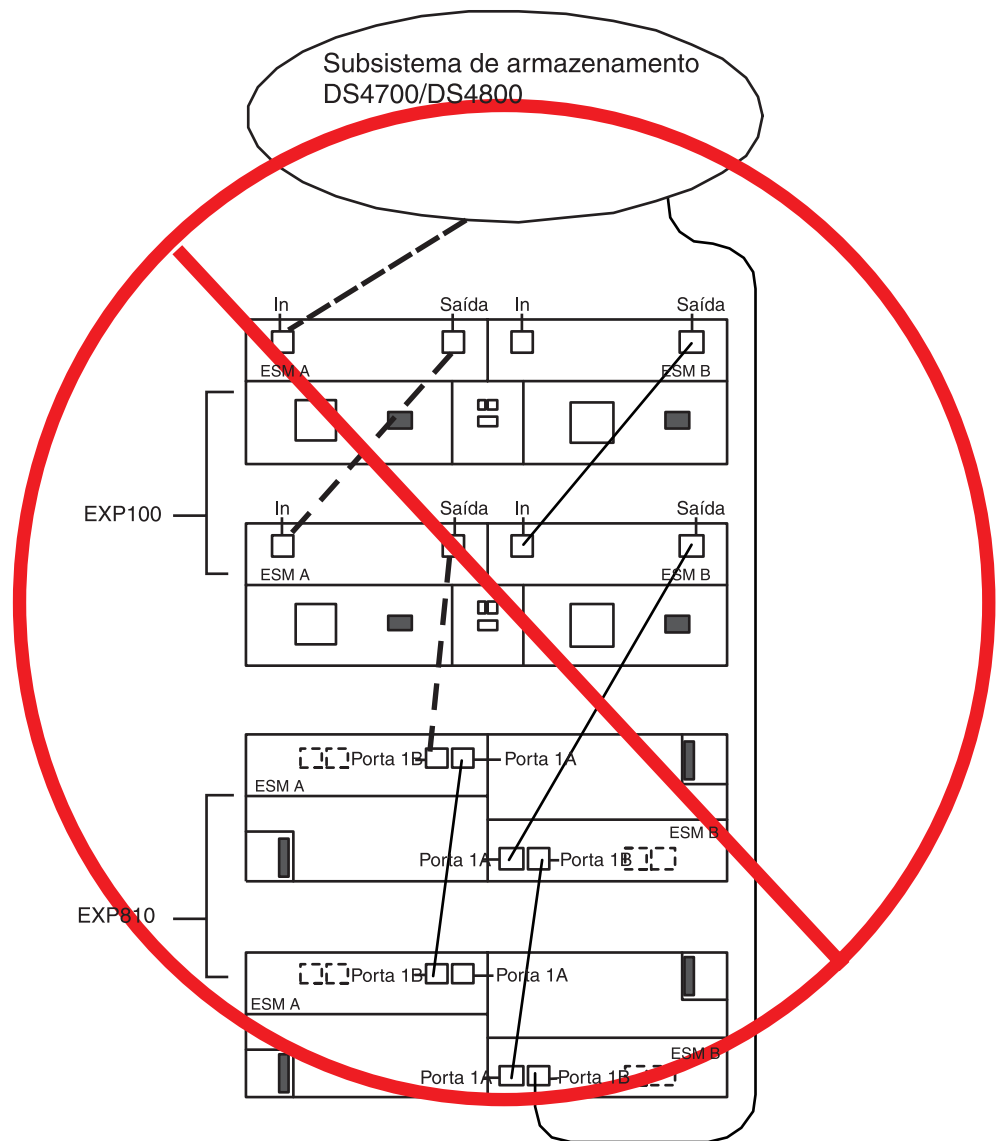
Figura 41. Configuração não suportada de intermistura de gabinete de armazenamento EXP710, EXP810 e EXP100 em um subsistema de armazenamento DS4700 ou DS4800
