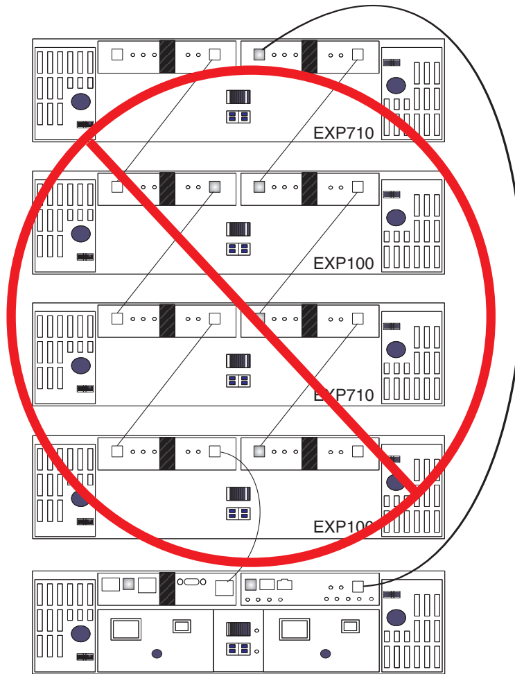
Figura 5. Configuração não suportada do loop do gabinete de armazenamento EXP100 e EXP710 (2 de 2)
