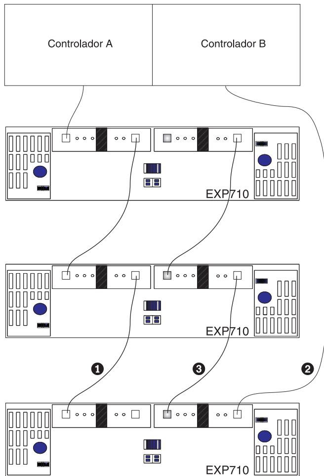
Figura 27. Cabeando um gabinete de armazenamento EXP700/EXP710/EXP100/EXP500 adicional
