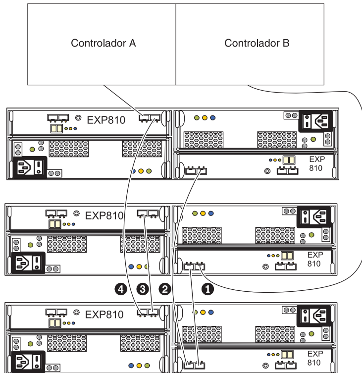
Figura 31. Cabeando um gabinete de armazenamento adicional para o meio do loop de unidade em um subsistema de armazenamento DS5000
