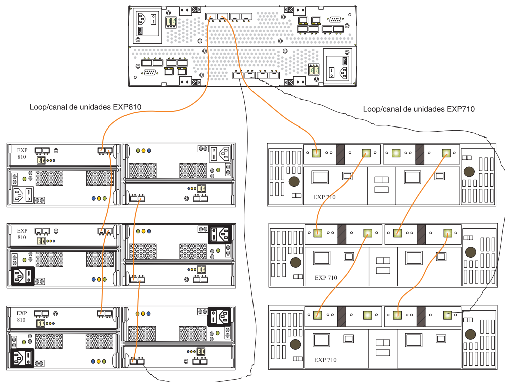
Figura 8. Subsistema de armazenamento DS4000 intermisturado recomendado conectado à configuração de loop de gabinete de armazenamento EXP710 e EXP810
