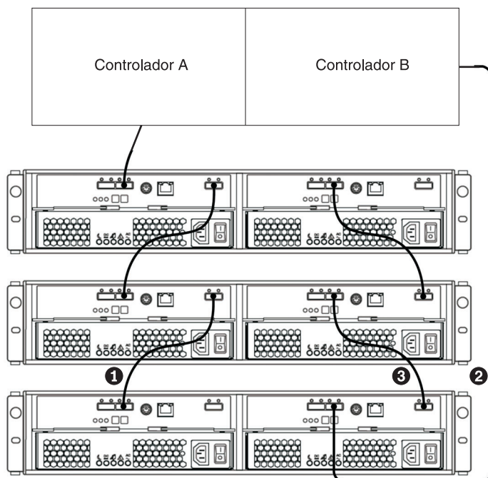
Figura 29. Cabeando um gabinete de armazenamento EXP3000, EXP3512 ou EXP3524 adicional
