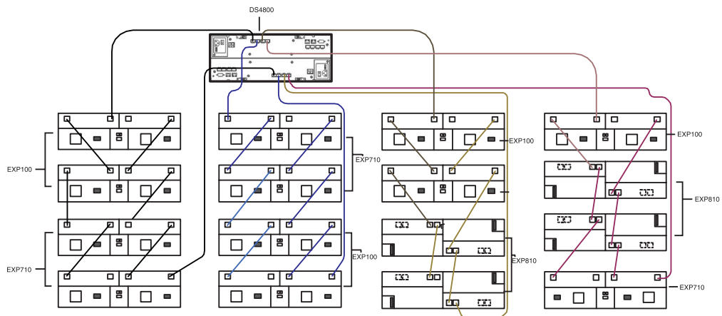
Figura 42. Variações de cabeamento quando os gabinetes de armazenamento EXP100, EXP710 e EXP810 estão intermisturados atrás de um subsistema de armazenamento DS4800
