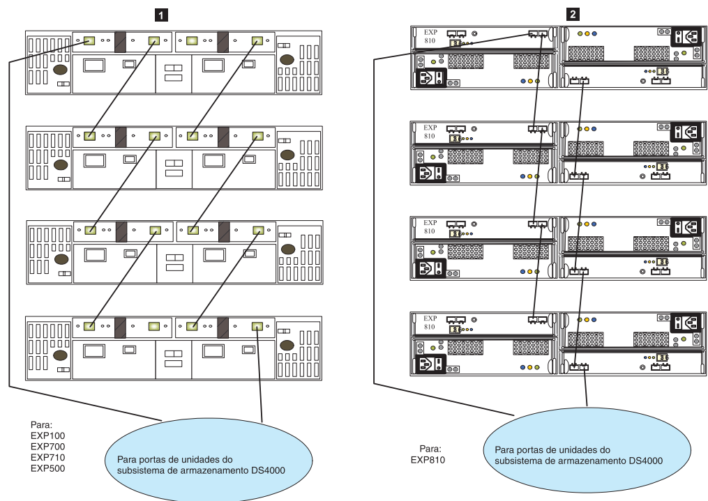
Figura 35. Melhor prática de esquema de loops de cabos para conexão de dispositivos de armazenamento
