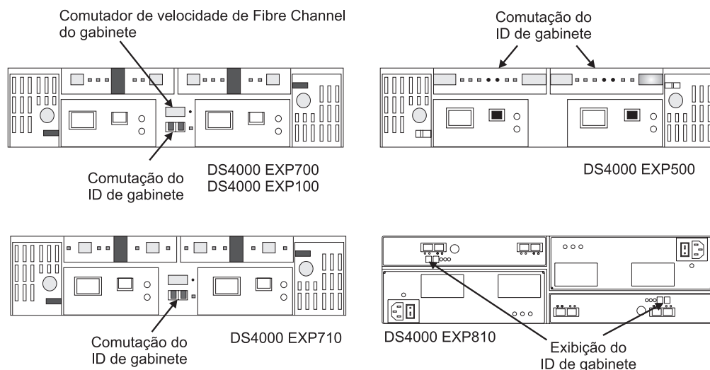
Figura 25. ID e comutadores de velocidade de gabinete de armazenamento EXP100, EXP500, EXP700, EXP710, EXP395/EXP420/EXP520/EXP810/EXP5000
