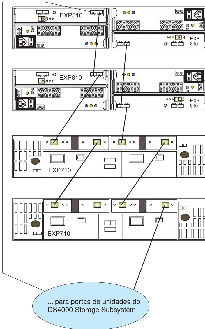
Figura 7. Subsistema de armazenamento DS4000 intermisturado suportado conectado à configuração de loop de gabinete de armazenamento EXP710 e EXP810
