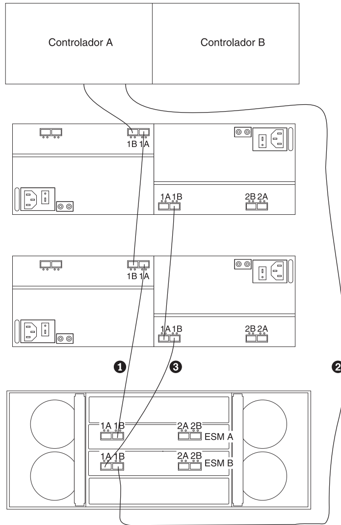
Figura 30. Cabeando um gabinete de armazenamento EXP5060 adicional
