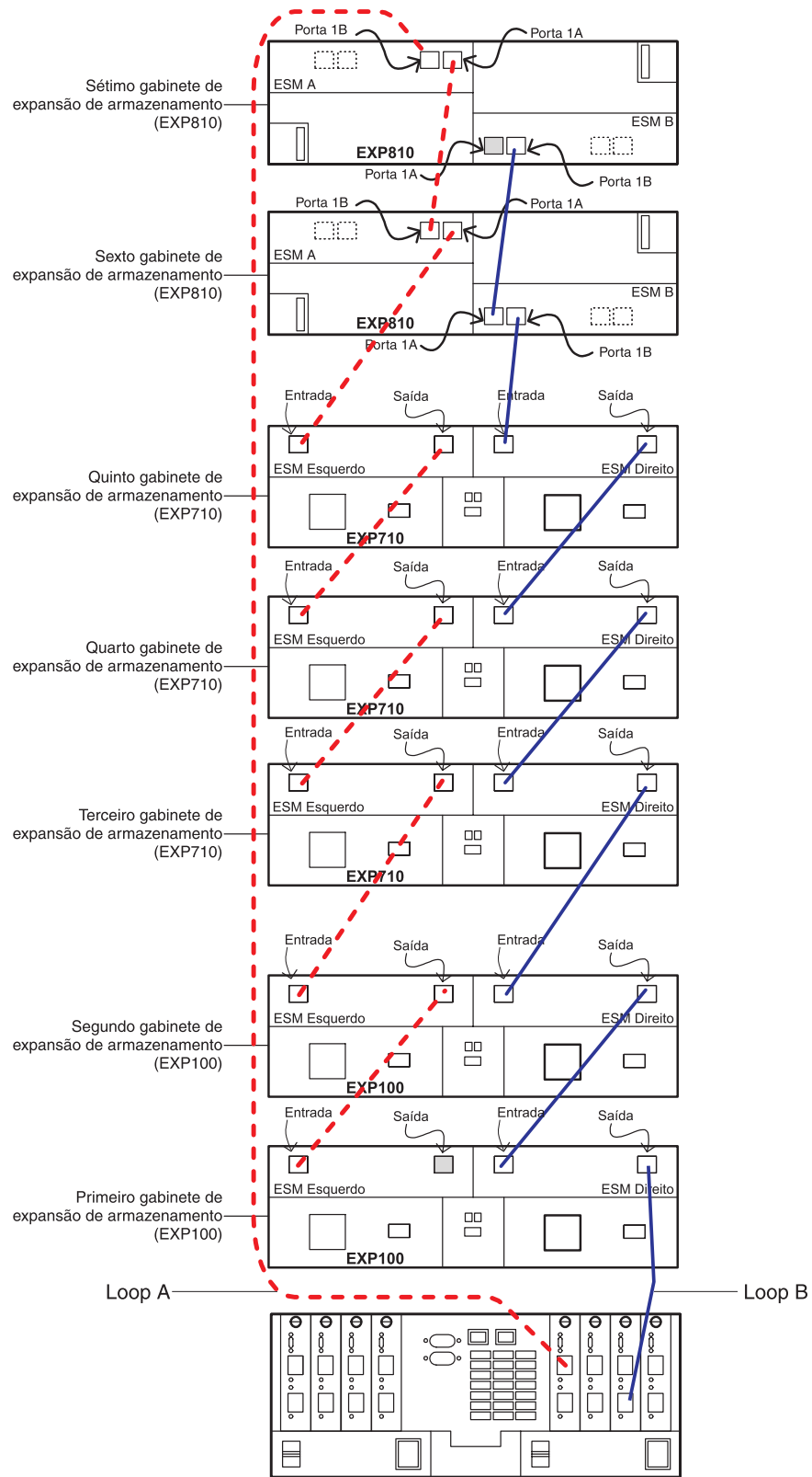
Figura 11. Cabeamento suportado para uma intermistura de gabinetes de armazenamento EXP100, EXP710 e EXP810 (exemplo 1)
