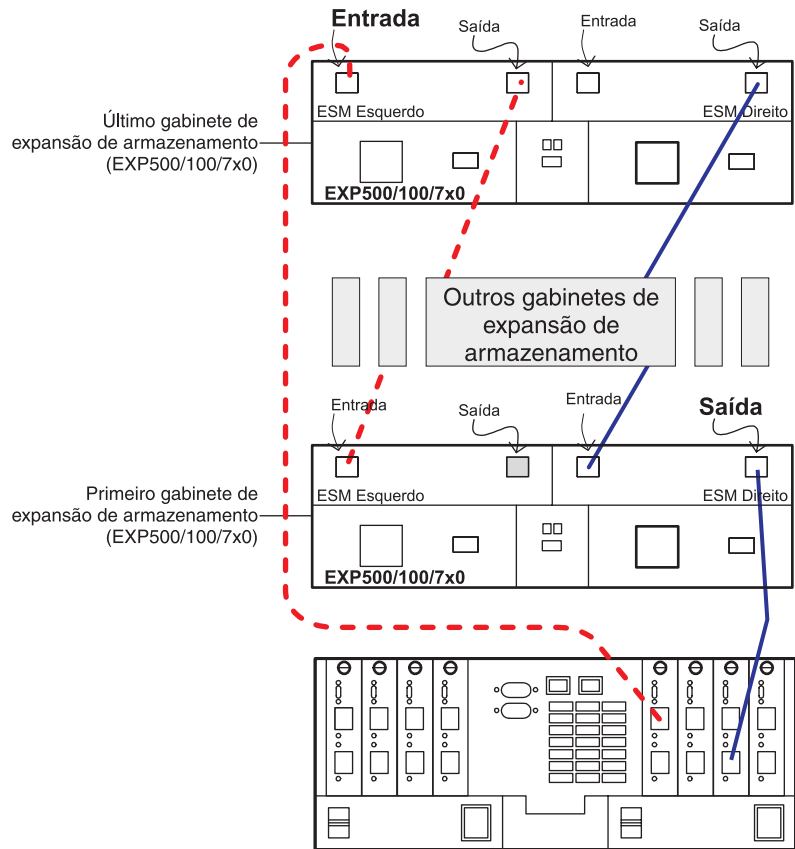
Figura 17. Cabeamento suportado para as portas do gabinete de armazenamento EXP500/EXP100/EXP700/EXP710
