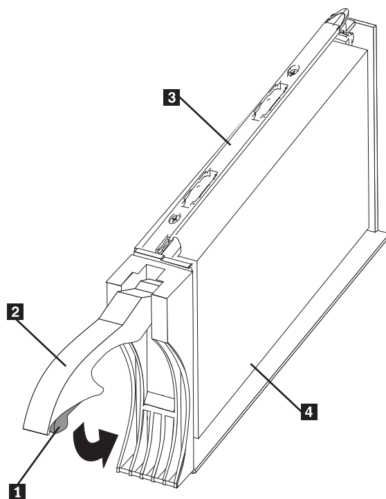
Figura 19. Montagem da CRU da Unidade
