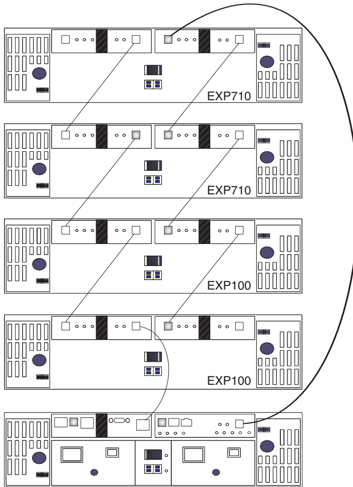
Figura 2. Configuração suportada do loop do gabinete de armazenamento EXP100 e EXP710 intermisturado (2 de 3)
