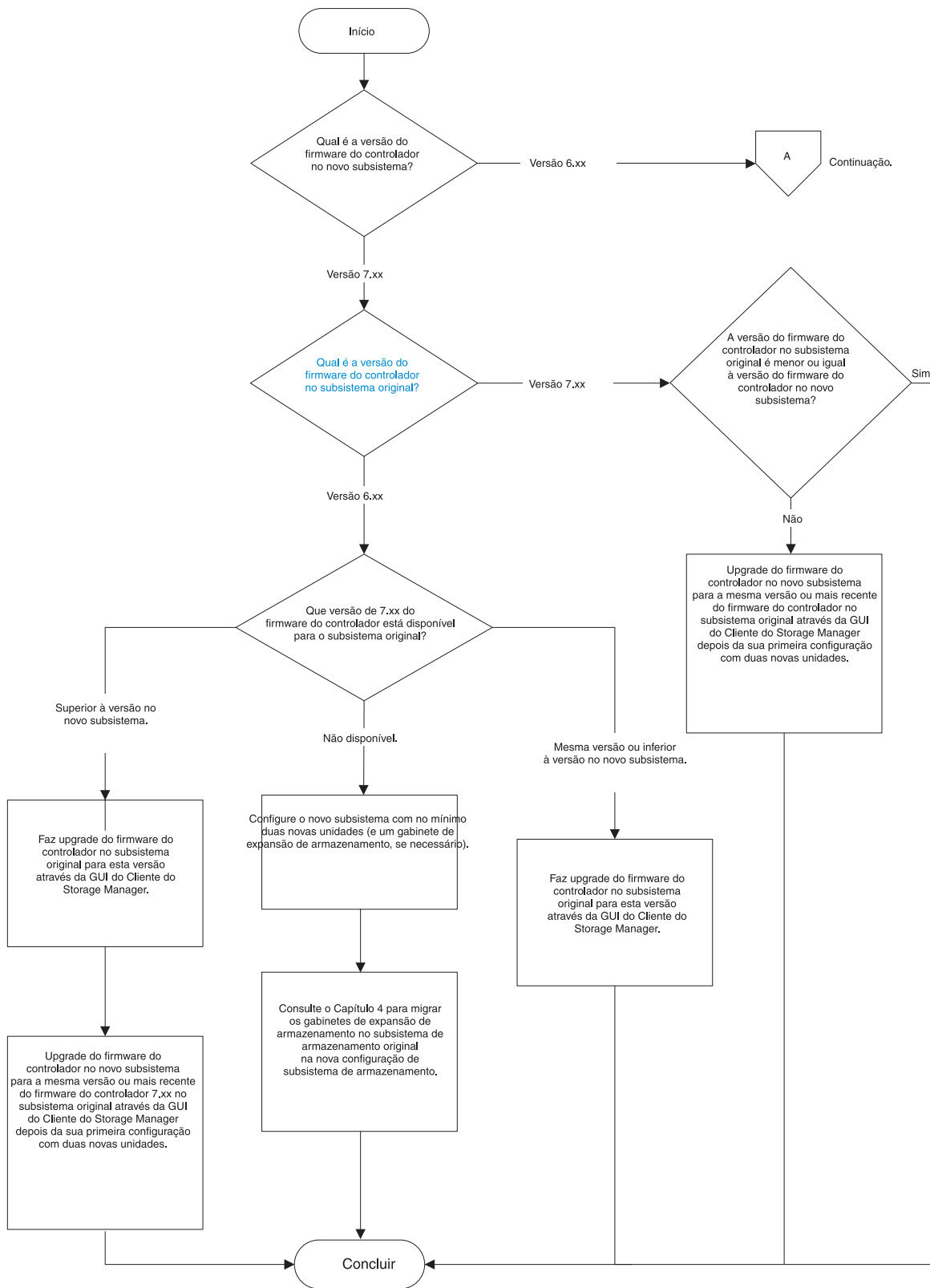
Figura 43. Fluxograma de compatibilidade de firmware para um upgrade do subsistema de armazenamento
