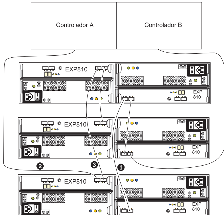
Figura 33. Cabeando um gabinete de armazenamento adicional para o início do loop de unidade em um subsistema de armazenamento DS5000
