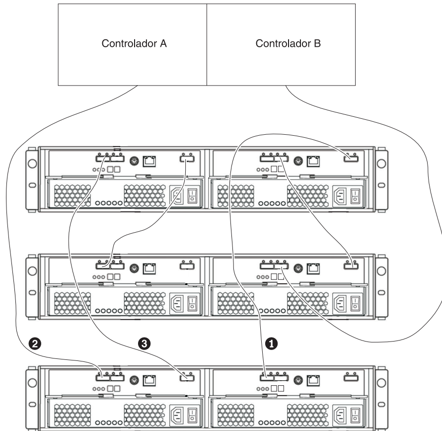
Figura 34. Cabeando um gabinete de armazenamento adicional para o início do loop de unidade em uma configuração do subsistema de armazenamento DS3000
