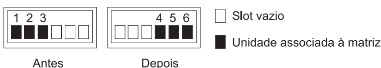
Figura 20. A melhor prática para reordenar uma matriz definida usando compartimentos vazios em um gabinete de armazenamento
