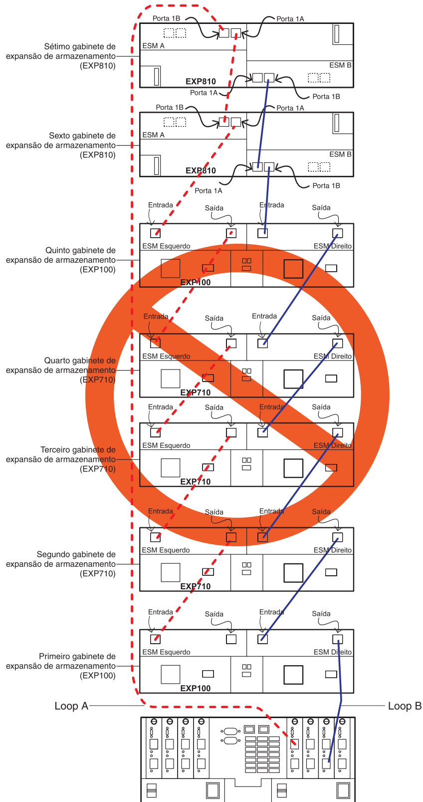
Figura 13. Cabeamento não suportado para uma intermistura de gabinetes de armazenamento EXP100, EXP710 e EXP810 (exemplo 1)
