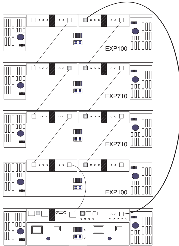
Figura 3. Configuração suportada, mas não recomendada, do loop do gabinete de armazenamento EXP100 e EXP710 intermisturado (3 de 3)
