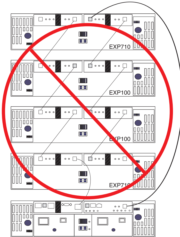
Figura 4. Configuração não suportada do loop do gabinete de armazenamento EXP100 e EXP710 (1 de 2)
