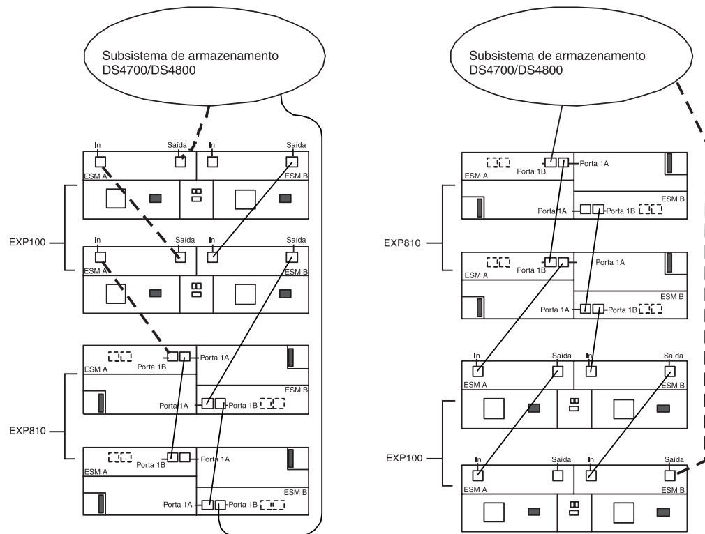
Figura 40. Configuração suportada de intermistura de gabinete de armazenamento EXP710, EXP810 e EXP100 em um subsistema de armazenamento DS4700 ou DS4800
