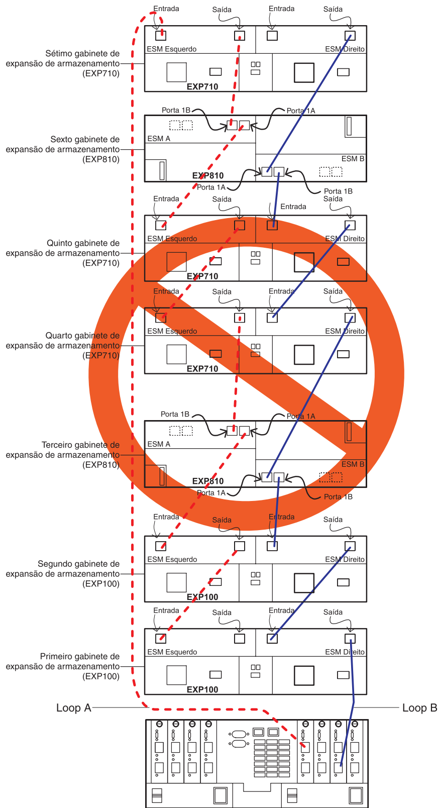
Figura 14. Cabeamento não suportado para uma intermistura de gabinetes de armazenamento EXP100, EXP710 e EXP810 (exemplo 2)
