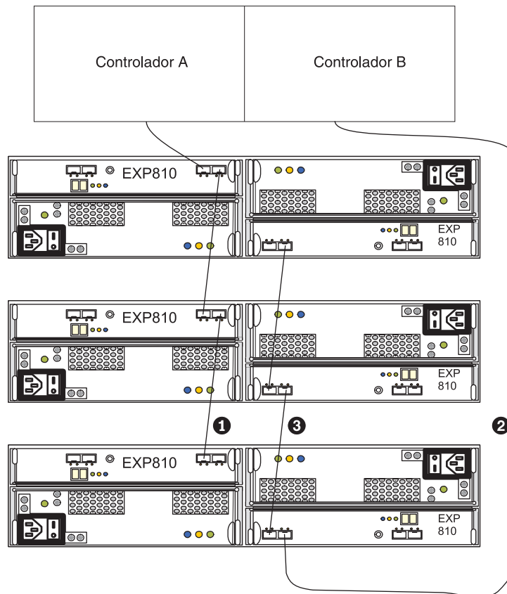
Figura 28. Cabeando um gabinete de armazenamento EXP5000, EXP520, EXP395, EXP810 ou EXP420 adicional
