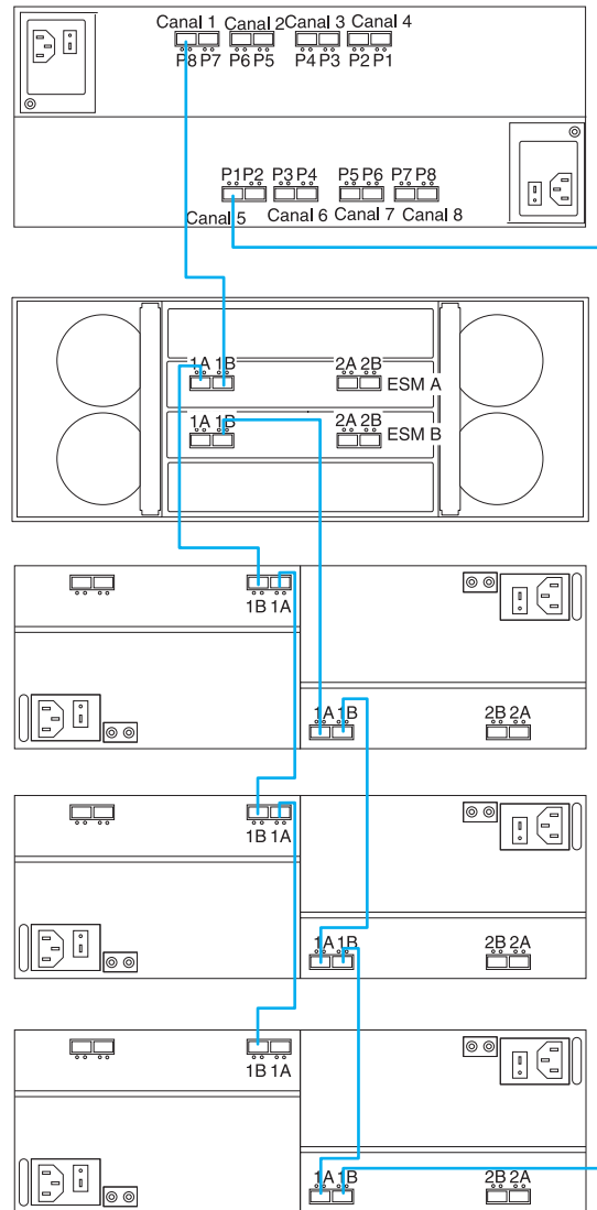
Figura 9. Configuração recomendada de cabo de unidade/loop de gabinete de armazenamento EXP5000 e EXP5060 intermisturado
