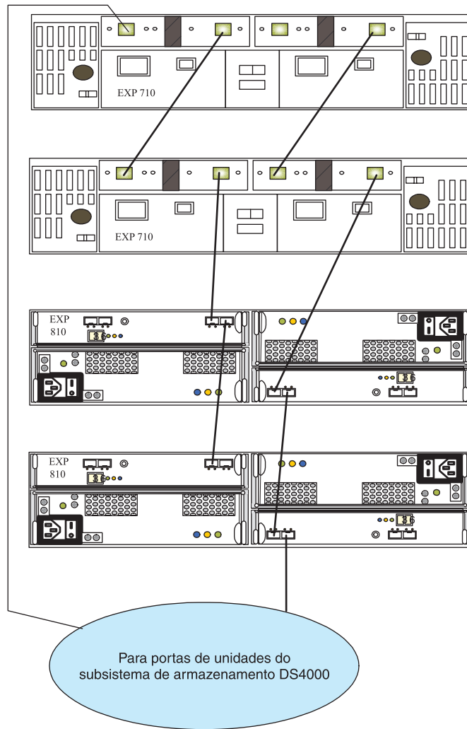
Figura 6. Subsistema de armazenamento DS4000 intermisturado suportado conectado à configuração de loop de gabinete de armazenamento EXP710 e EXP810
