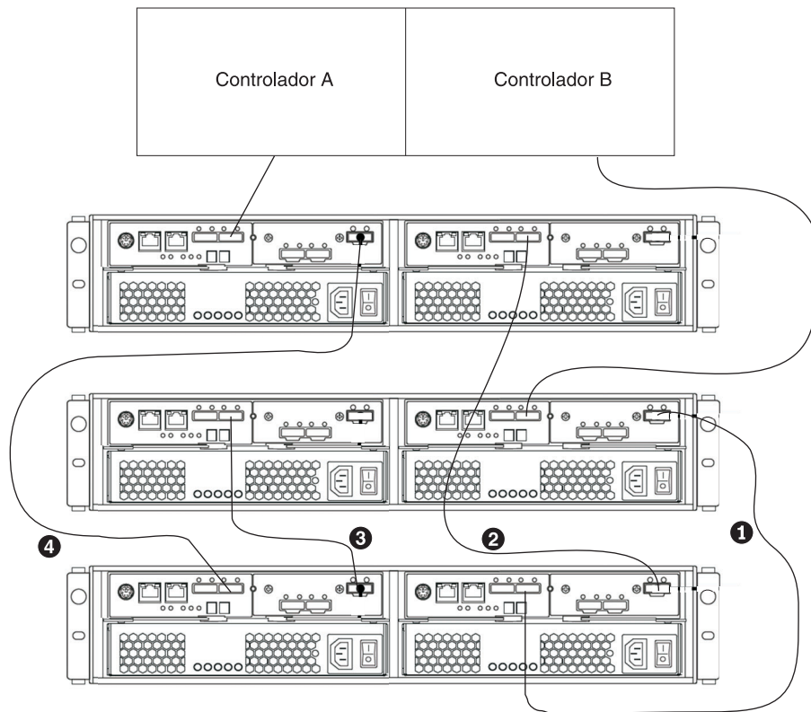
Figura 32. Cabeando um gabinete de armazenamento adicional para o meio do loop de unidade em uma configuração do subsistema de armazenamento DS3000
