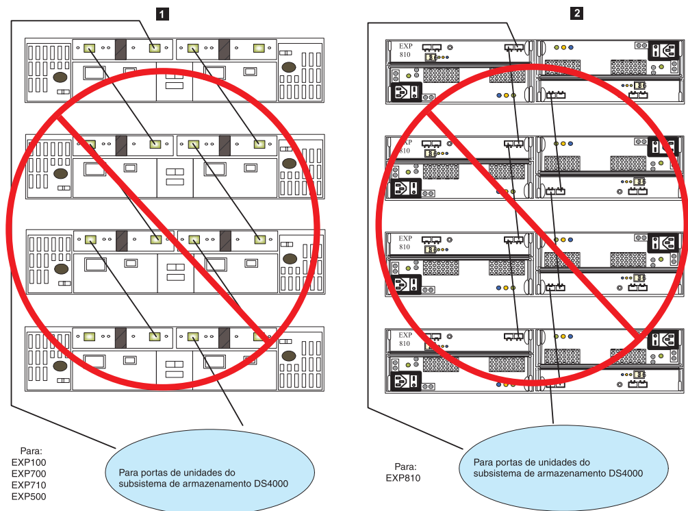
Figura 36. Esquema alternativo de loops de cabos para conexão de dispositivos de armazenamento
