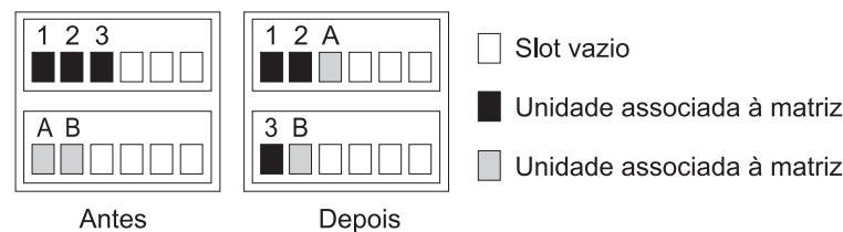
Figura 22. Reordenando múltiplas matrizes definidas nos compartimentos anteriormente usados em dois gabinetes de armazenamento
