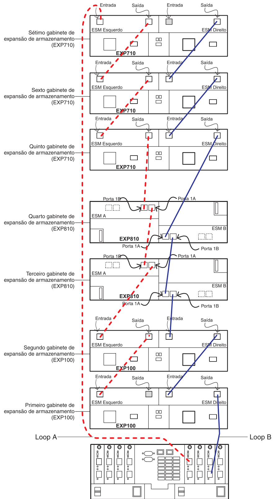
Figura 12. Cabeamento suportado para uma intermistura de gabinetes de armazenamento EXP100, EXP710 e EXP810 (exemplo 2)
