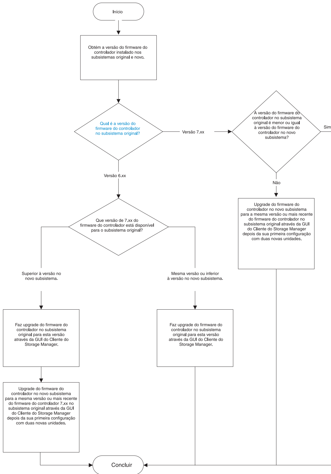
Figura 45. Fluxograma de compatibilidade de firmware para upgrade de um DS4700 ou DS4800 para um subsistema de armazenamento DS5000
