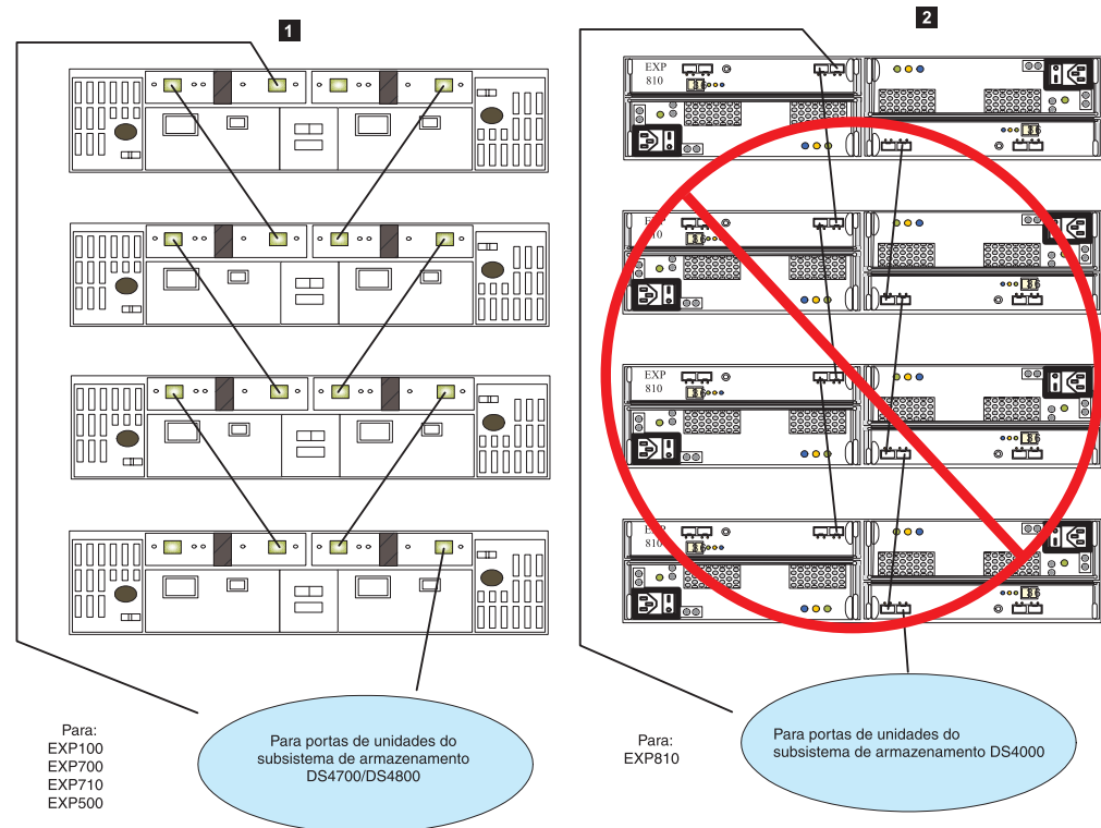
Figura 37. Esquema alternativo de loops de cabos para conexão de dispositivos de armazenamento
