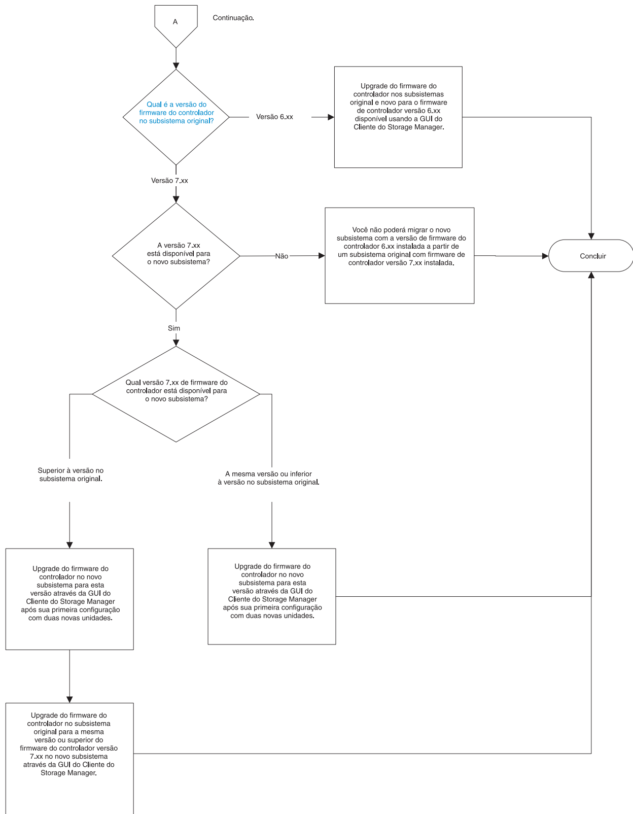
Figura 44. Fluxograma de compatibilidade de firmware para um upgrade do subsistema de armazenamento (continuação)
