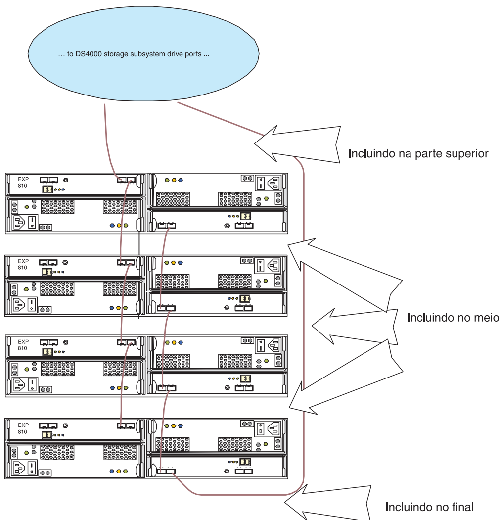
Figura 26. Exemplo de inclusão de posições do gabinete de armazenamento em um loop de unidade
