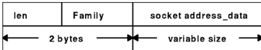
sockaddr Structure
